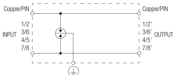
modello S-F 1/48 PoE+ b Cod. 318 010 schema di principio per ognuna delle quattro coppie di fili di ogni linea
