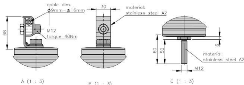
Installazione terminale di terra
