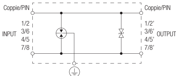
modello S-F 1/6 Cod. 318 008 schema di principio per ognuna delle quattro coppie di fili di ogni linea
