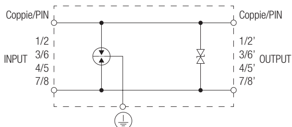
modello S-F 1/48 PoE+ Cod. 318 009 schema di principio per ognuna delle quattro coppie di fili di ogni linea
